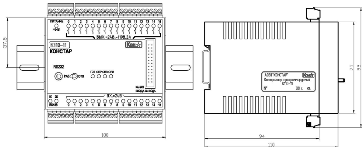
Рисунок 1.3. Габаритные и установочные размеры базового блока К110
