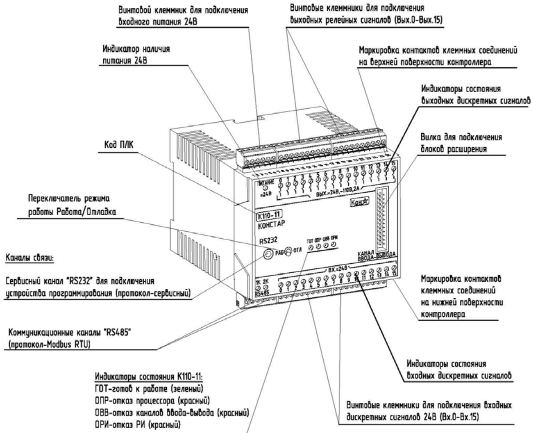
Рисунок 1.2. Внешний вид типового базового блока К110
